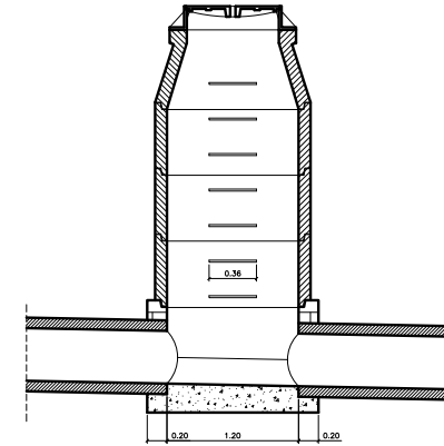
SECCIO B-B' escala = 1 : 40
