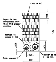
2 CIRCUITS EN TERRA
