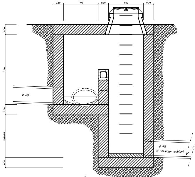
SECCIO A-A' escala = 1 : 40
