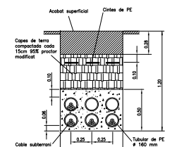
4 CIRCUITS EN CALÇADA (CREUAMENTS)
