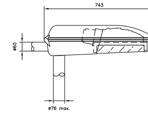
SECCIÓ LONGITUDINAL
