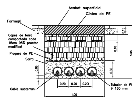
4 CIRCUITS EN VORERA (QUAL NORMAL)
