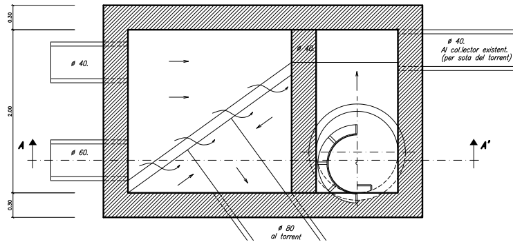
PLANTA SOBREGIDOR 2. escala = 1 : 40
