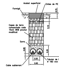
2 CIRCUITS EN VORERA
