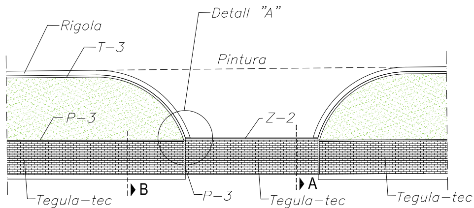
Detall Accés
