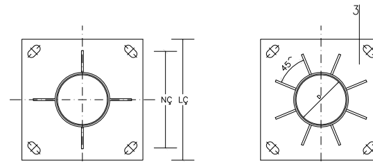
SECCIÓ BASE H = 7.5 / 9 / 10 m
