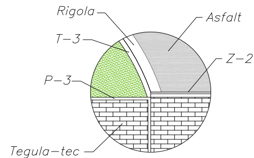
Detall "A"
