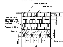
4 CIRCUITS EN TERRA
