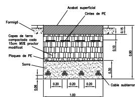
4 CIRCUITS EN VORERA
