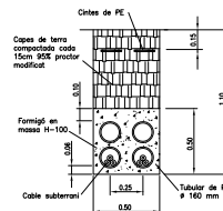
2 CIRCUITS EN TERRA (QUAL REFORÇAT)
