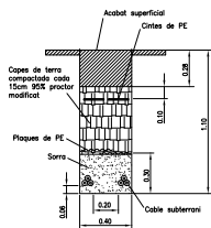
2 CIRCUITS EN CALÇADA
