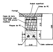
2 CIRCUITS EN FORMIGÓ
