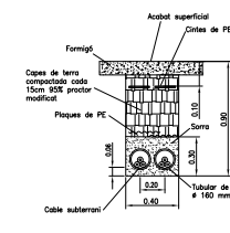
2 CIRCUITS EN FORMIGÓ
