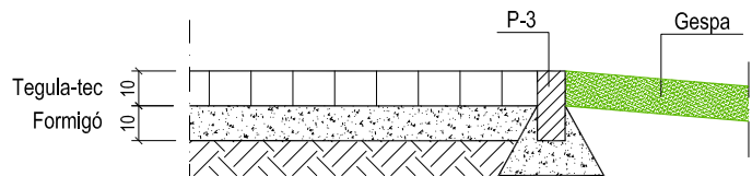
Secció B
