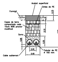
2 CIRCUITS EN VORERA
