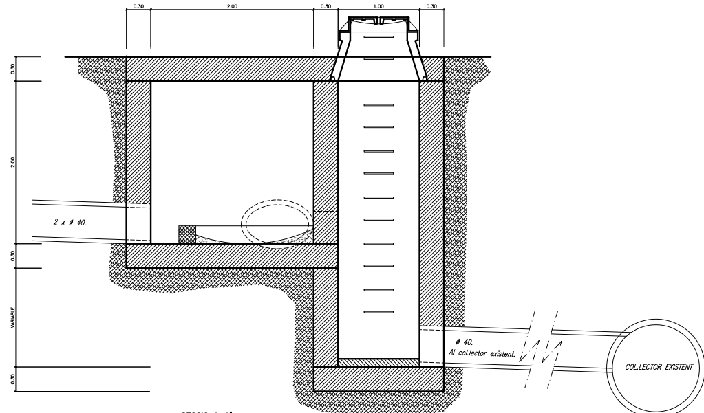
SECCIO A-A' escala = 1 : 40
