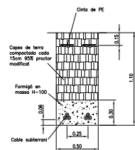
2 CIRCUITS EN TERRA
