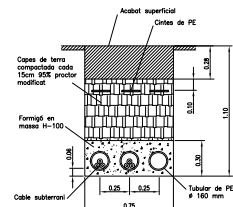
2 CIRCUITS EN CALÇADA (CREUAMENTS)
