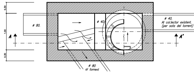
PLANTA SOBREGIDOR 1. escala = 1 : 40
